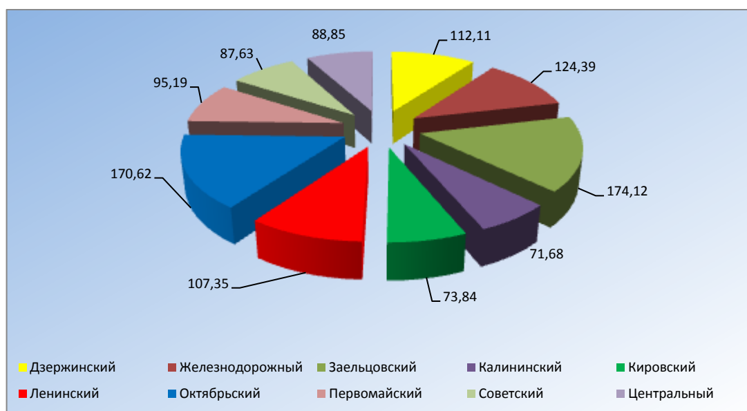
Рисунок 1.5 – Объем ТБО, образующихся на территории инфраструктуры, тыс. м 3 .
