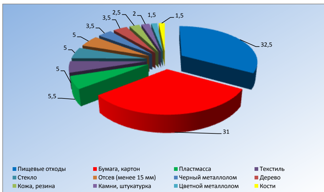
Рисунок 1.7 – Морфологический состав ТБО, образующихся на территории города Новосибирска, %
