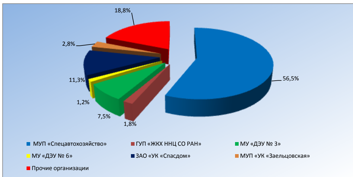
Рисунок 2.1 – Доли рынка вывоза ТБО в г. Новосибирске, %
