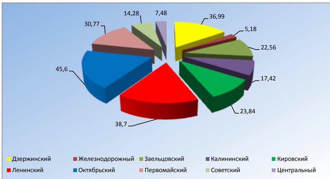
Рисунок 1.4 – Объем ТБО, образующихся на территории жилищного фонда частного сектора, тыс. м 3 .
