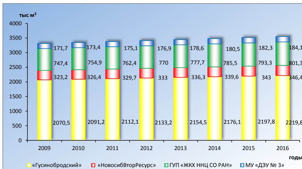
Рисунок 1.2 – Динамика распределения ТБО по полигонам
