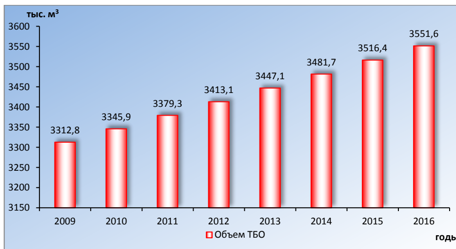
Рисунок 1.1 – Динамика поступления ТБО на полигоны Новосибирска
