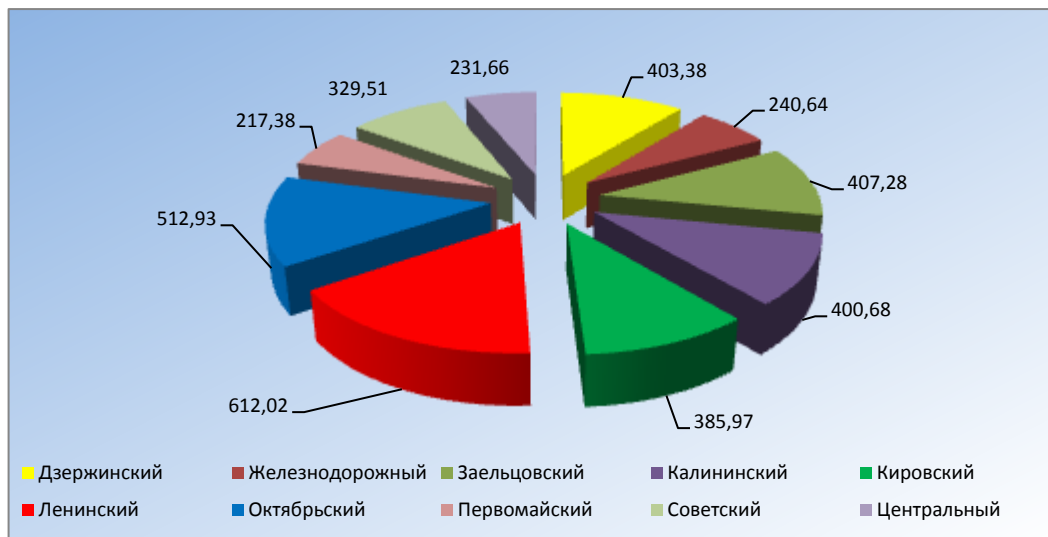
Рисунок 1.6 – Суммарный объем ТБО по районам г. Новосибирска, тыс. м 3 .
