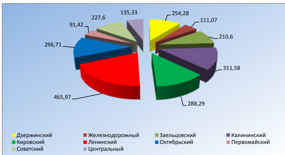
Рисунок 1.3 – Объем ТБО, образующихся на территории жилищного фонда многоквартирных домов, тыс. м 3 .
